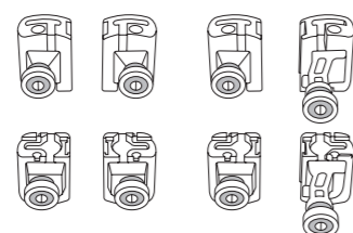
Millenium Nisch N3d (8 st) N3d höger = ingång höger sida utifrån N3d vänster = ingång vänster sida utifrån
