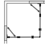
GRACE SPECIAL 2 Grace 2 DSL2, höjd 200 cm, måttbeställs mot förfrågan Max mått 170 X 170 cm.
