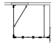
GRACE SPECIAL 16 Grace 16 DSL16, glashöjd 200cm. Max mått 100x220 cm.
