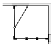
GRACE SPECIAL 15 Grace 15 DSL15, glashöjd 200cm. Max mått 100x150 cm.
