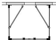
GRACE SPECIAL 13 Grace 13 DSL13, glashöjd 200cm. Max mått 100x100 cm.
